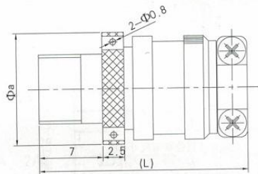
Y8C-nZJL(Z1JL)(ZKL)外形图
