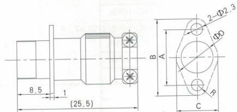
Y8C-nZJB1L(ZKB1L)外形及安装开口尺寸图
